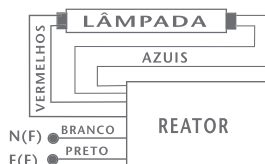
Esquema de ligação
